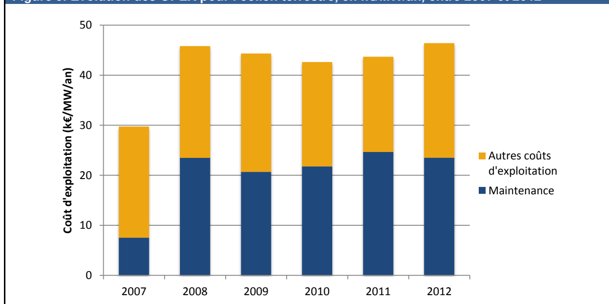
Figure 9. Évolution des OPEX pour l'éolien terrestre, en k€/MW/an, entre 2007 et 2012
